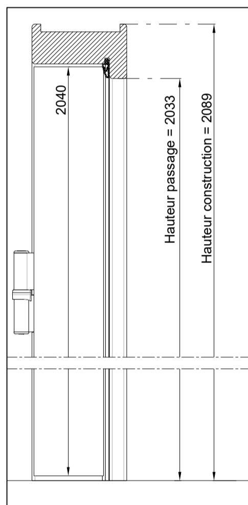
Coupe B-B' - Echelle 1/4
