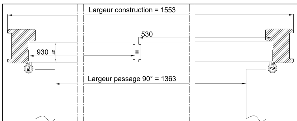
Coupe A-A' - Echelle 1/4
