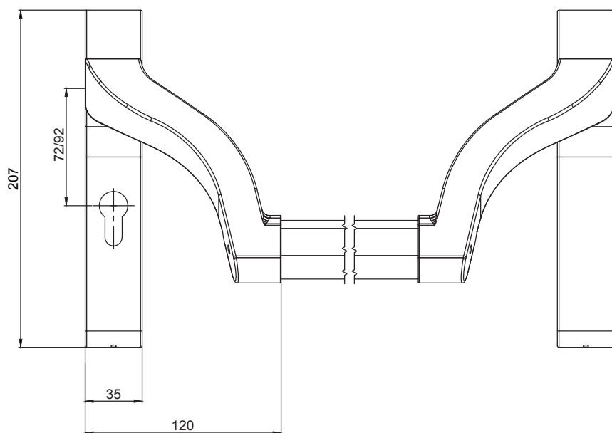
→ vue générale et dimensions
