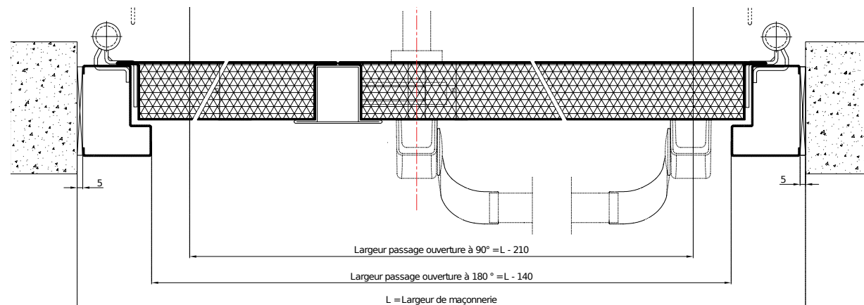
Coupe 2 vantaux
