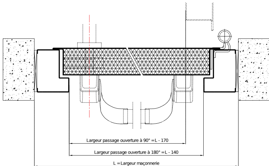
Coupe 1 vantail
