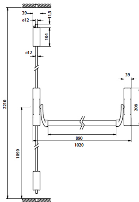
Barre antipanique Type PUSH 3 points en applique.
